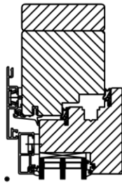
DETAIL E MABSTAB 1 : 5
