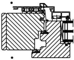
DETAIL C MABSTAB 1 : 5
