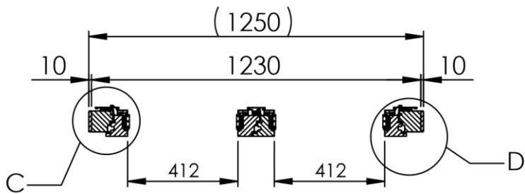
SCHNITT A-A
