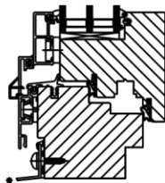
DETAIL F MABSTAB 1 : 5
